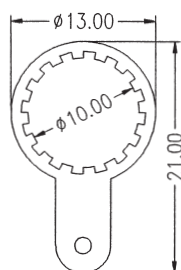
P/N RFA5-04 GROUNDING LUG
