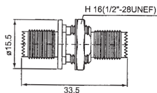
MU588CU-XNGD50 MINI UHF DOUBLE FEMALE BULKHEAD TYPE
