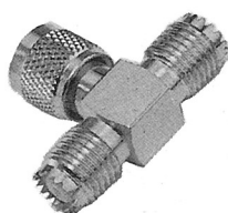
MU556CU-X***50 MINI UHF MALE TO MINI UHF DOUBLE FEMALE
