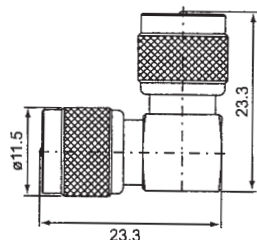
MU586CU-XNGD50 MINI UHF DOUBLE MALE RIGHT ANGLE TYPE
