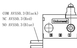
(G) Left Wire
