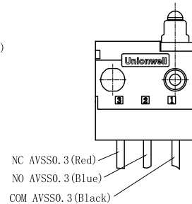
(E) Bottom Wire
