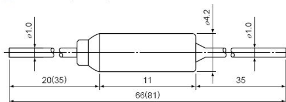
■ Dimension (Unit:mm)
