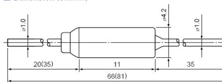
■ Dimension (Unit:mm)
