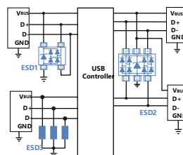
USB 2.0保护
