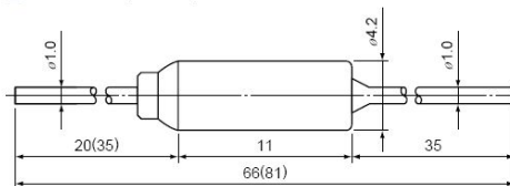
Dimension (Unit:mm)
