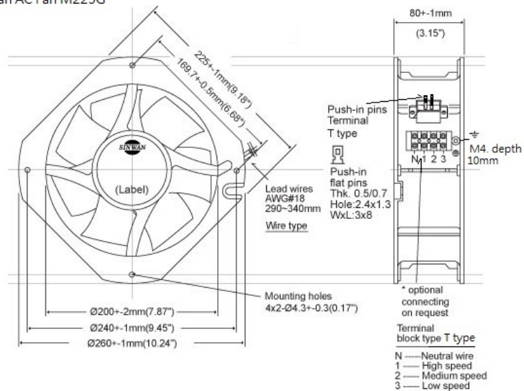
Sinwan AC Fan M225G
