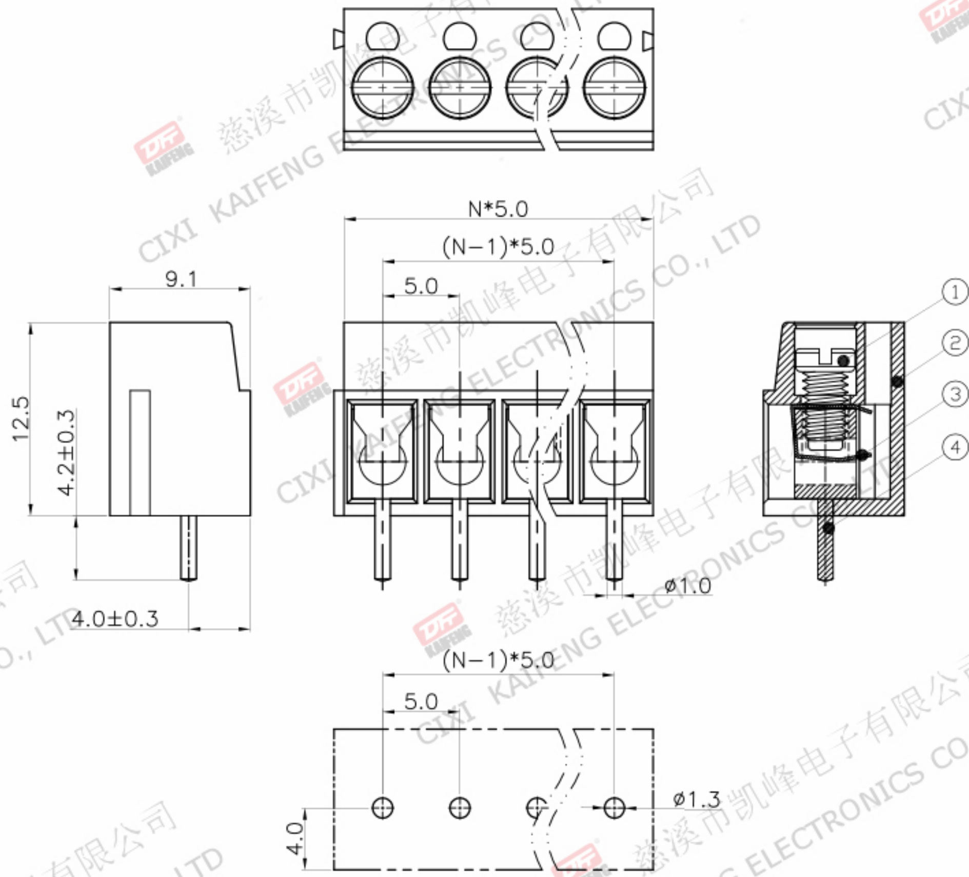
P.C.B.LAYOUT
