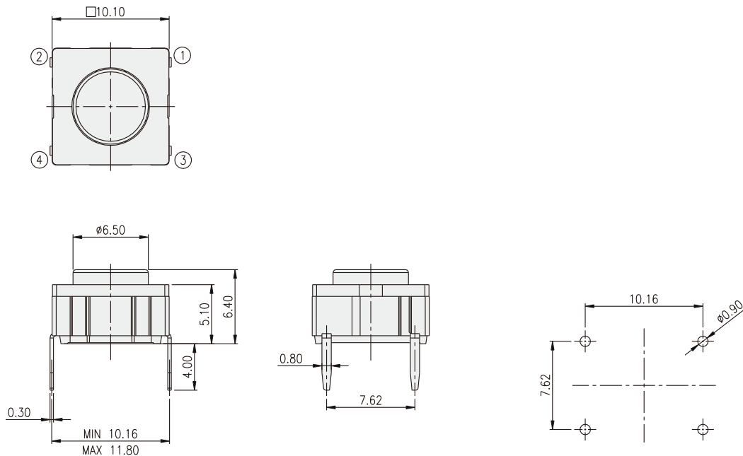
P.C.B. LAYOUT
